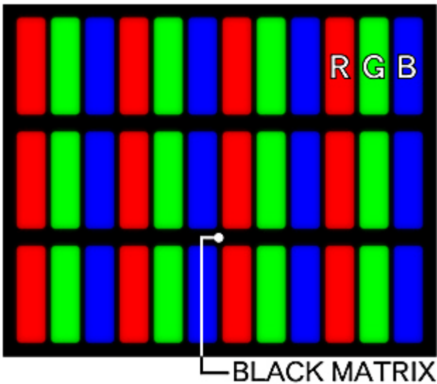
図 カラーフィルター概略図
